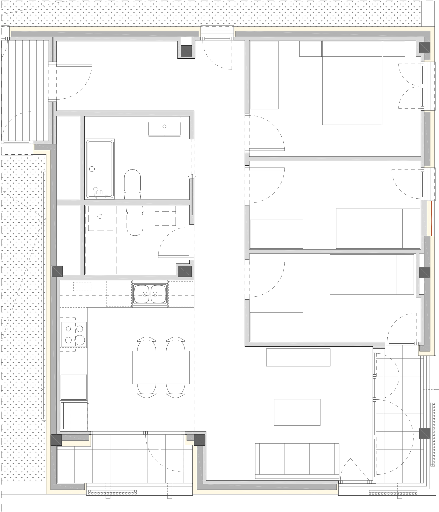
HABITATGE 5è 1a (HS7) Total Sup. Útil: 72,15 m 2 Total Sup. Construïda: 93,03 m 2
