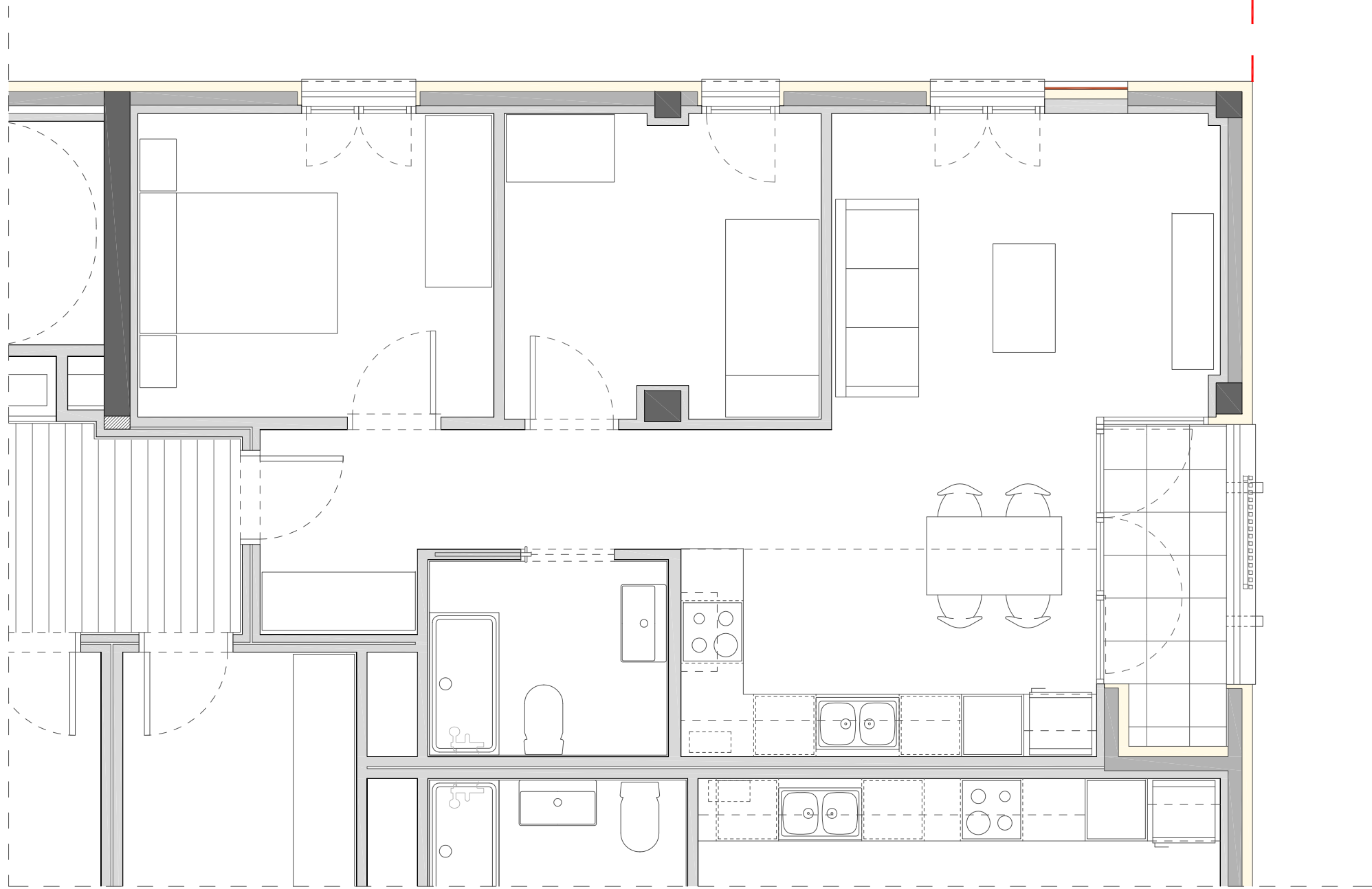
HABITATGE 1r 1a (HS5) Total Sup. Útil: 54,57 m 2 Total Sup. Construïda: 66,59 m 2
