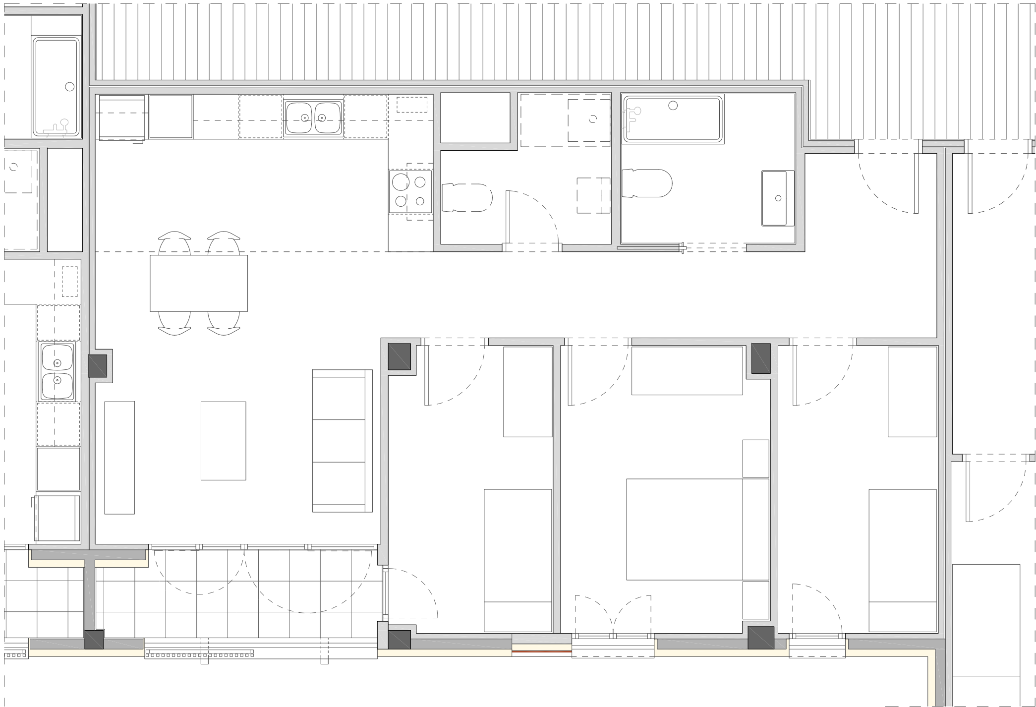
HABITATGE 2n 3a (HS3) Total Sup. Útil: 72,65 m² Total Sup. Construïda: 85,15 m²
