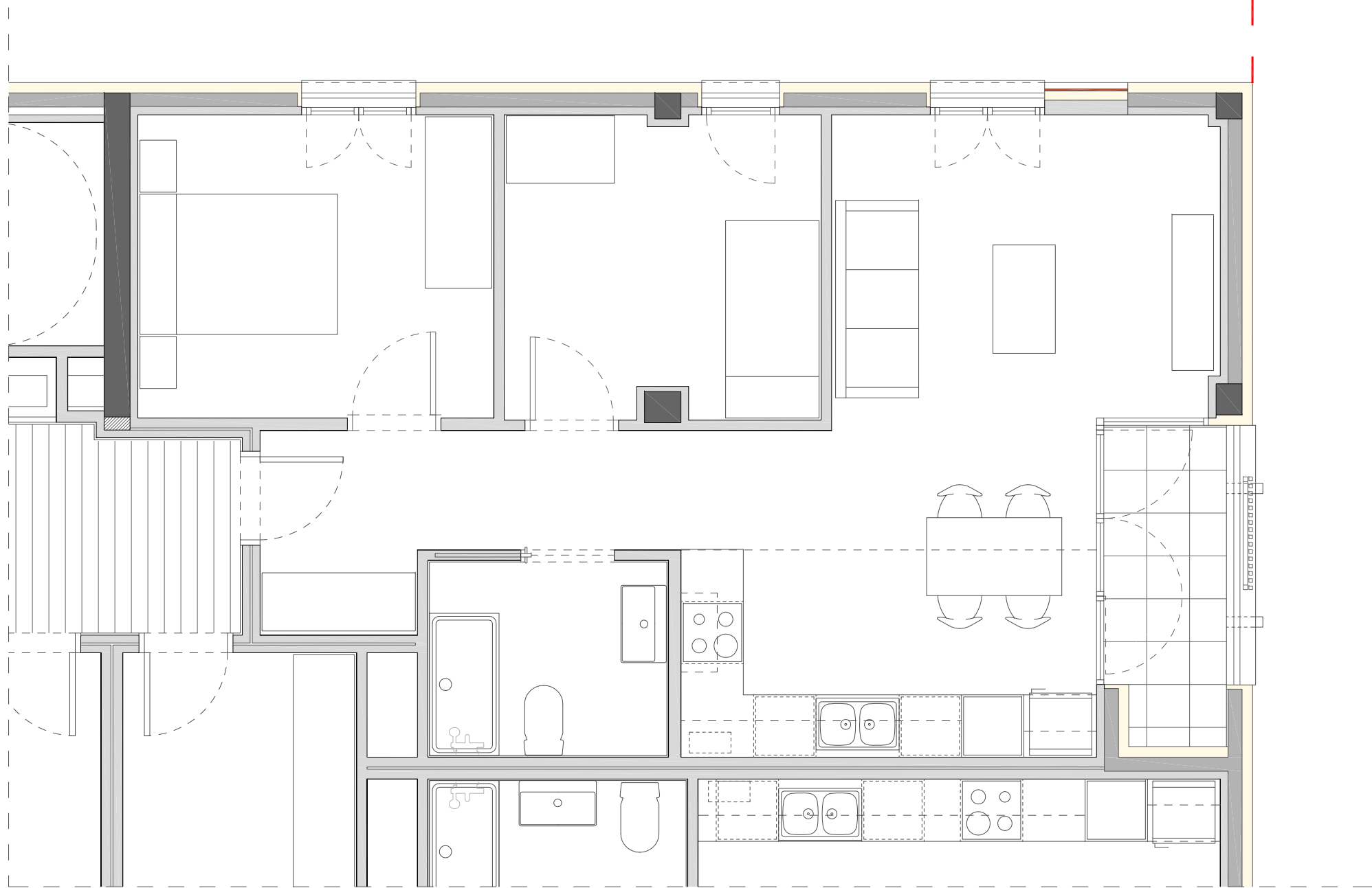
HABITATGE 3r 1a (HS5) Total Sup. Útil: 54,57 m 2 Total Sup. Construïda: 66,59 m 2
